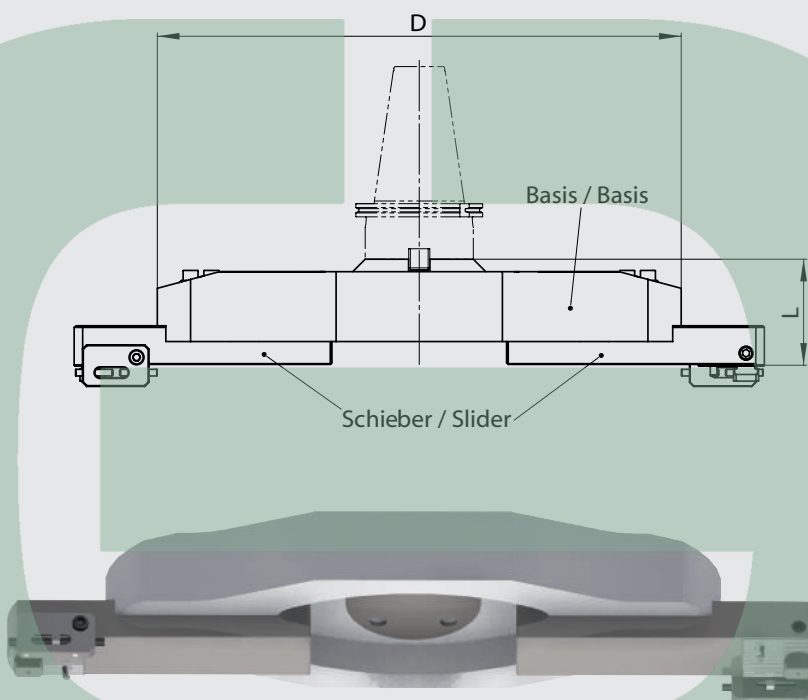
Aufnahmedorn für Verlängerungskonsolen
